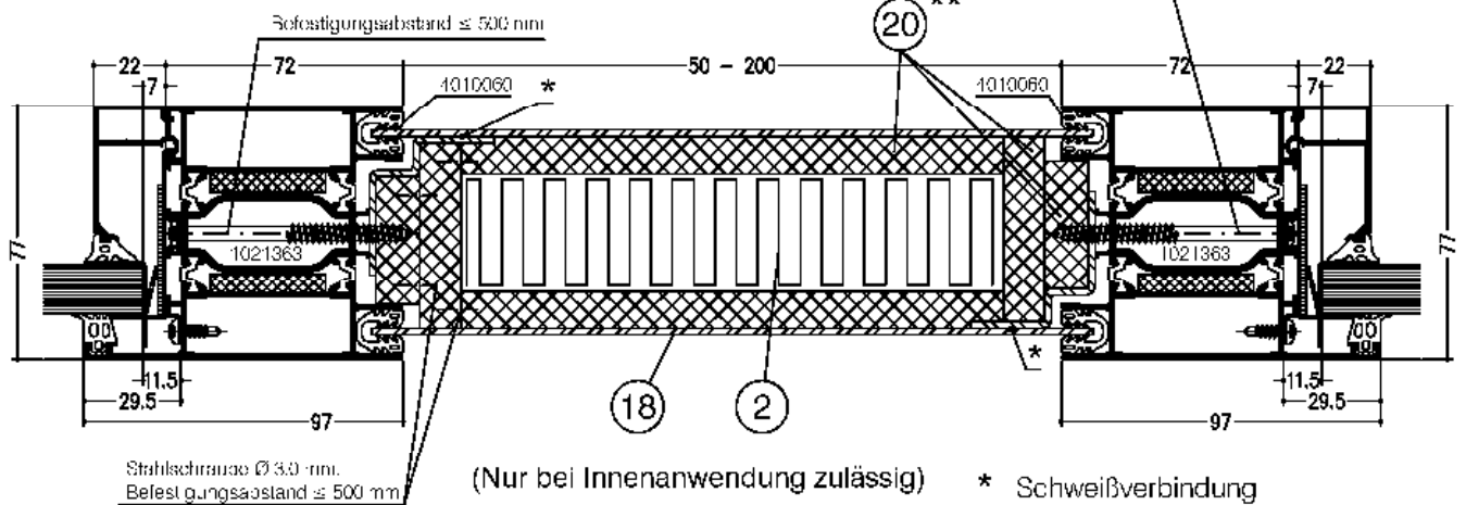
E-E (Ausfüllung Typ B)
