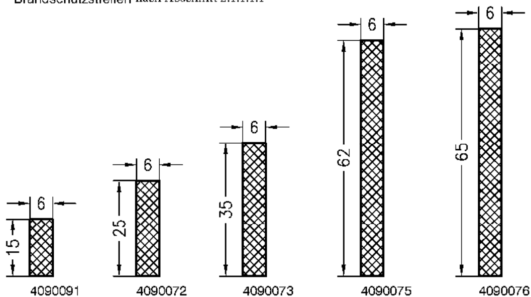
Brandschutzstreifen nach Abschnitt 2.1.1.1.1
